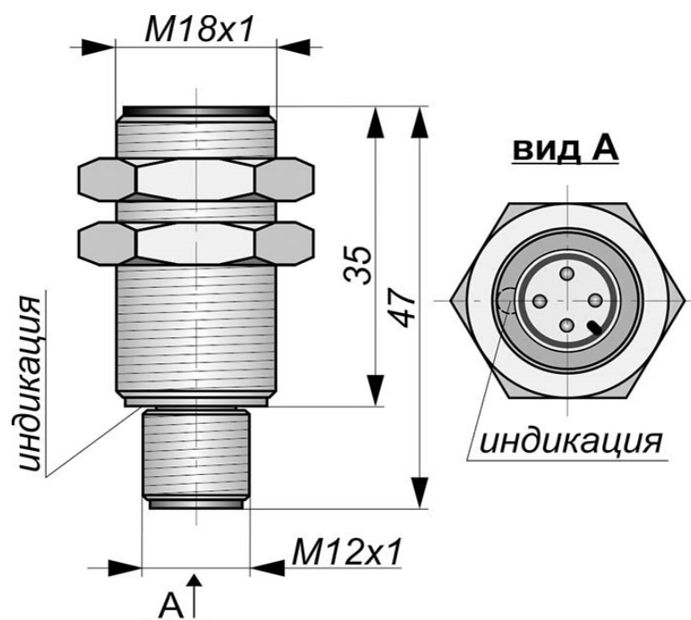
Габаритный чертеж
