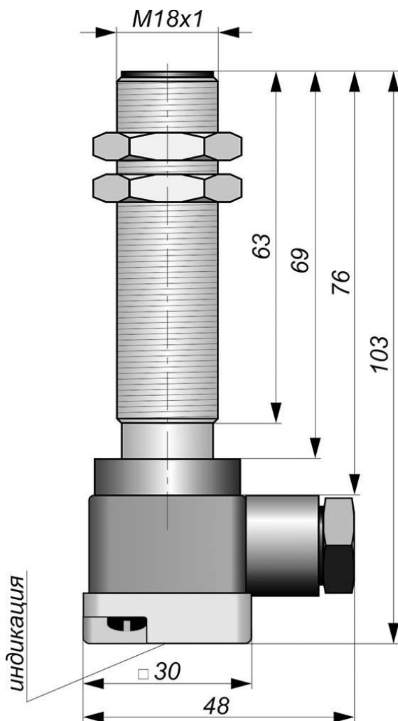
Габаритный чертеж
