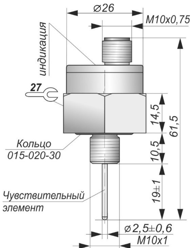
Габаритный чертеж
