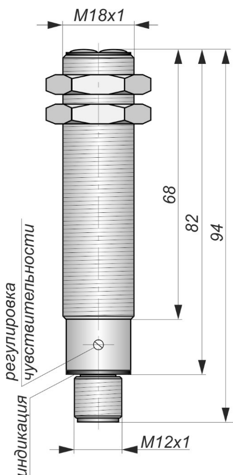
Габаритный чертеж
