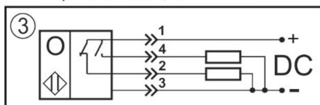
Переключающий контакт
