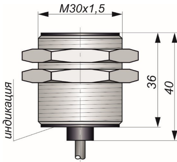
Габаритный чертеж
