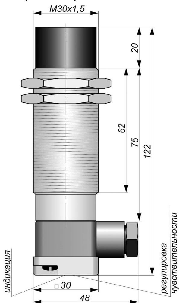
Габаритный чертеж
