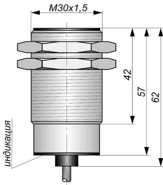
Габаритный чертеж
