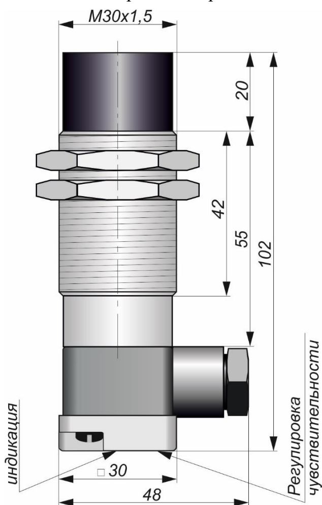
Габаритный чертеж
