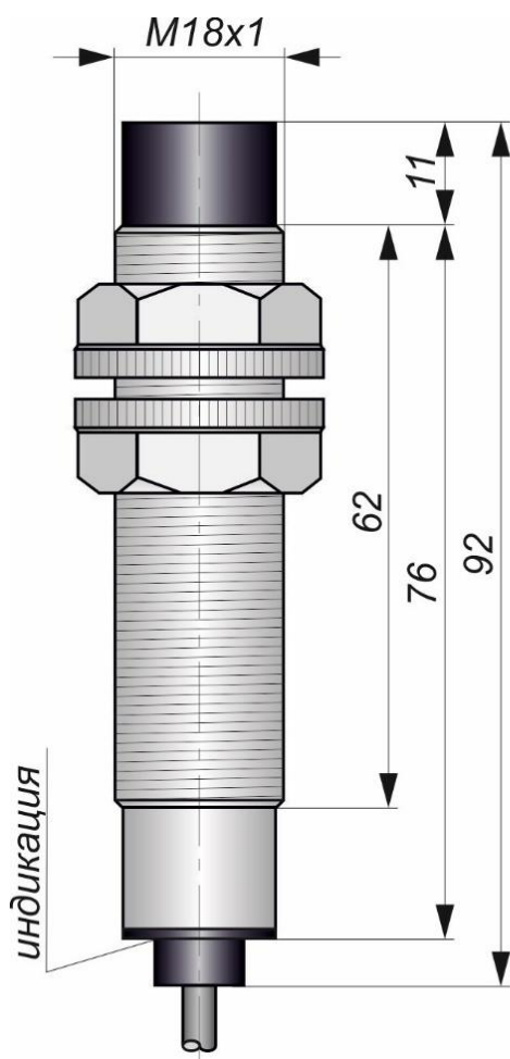
Габаритный чертеж
