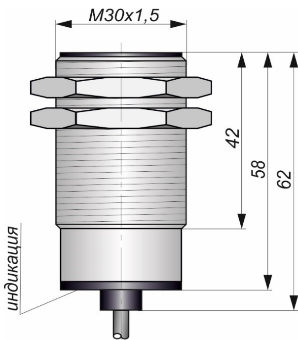
Габаритный чертеж
