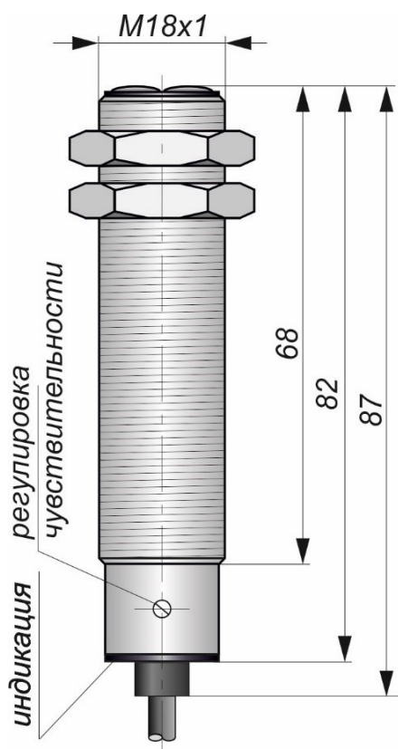
Габаритный чертеж
