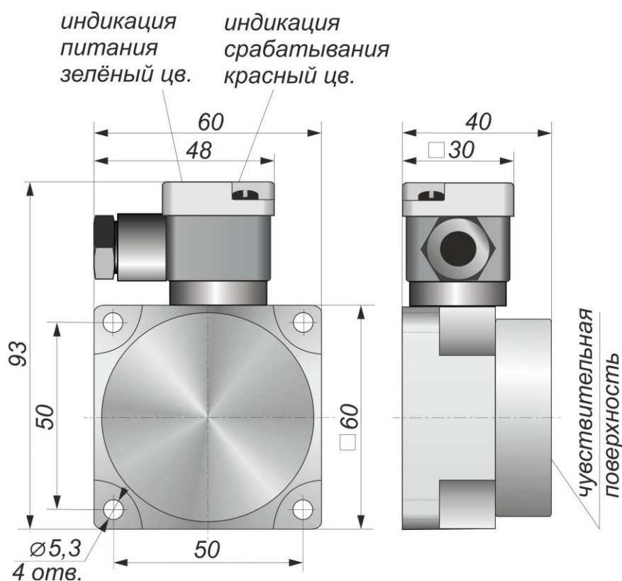
Габаритный чертеж
