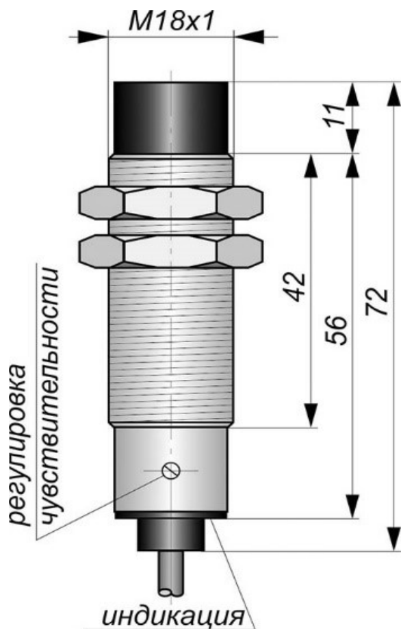
Габаритный чертеж
