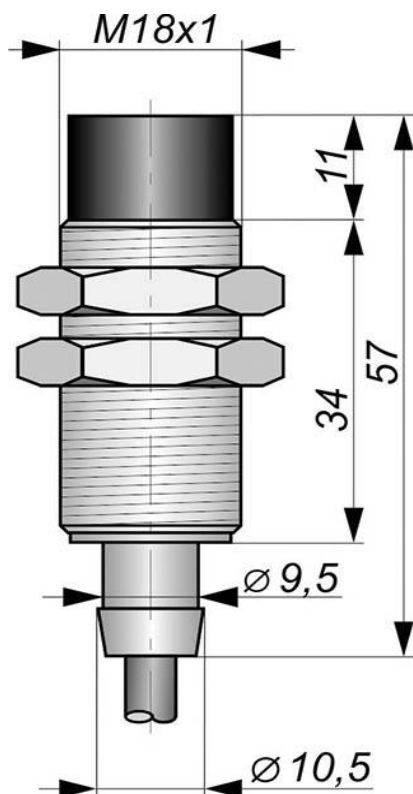
Габаритный чертеж
