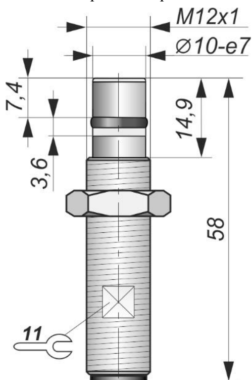
Габаритный чертеж
