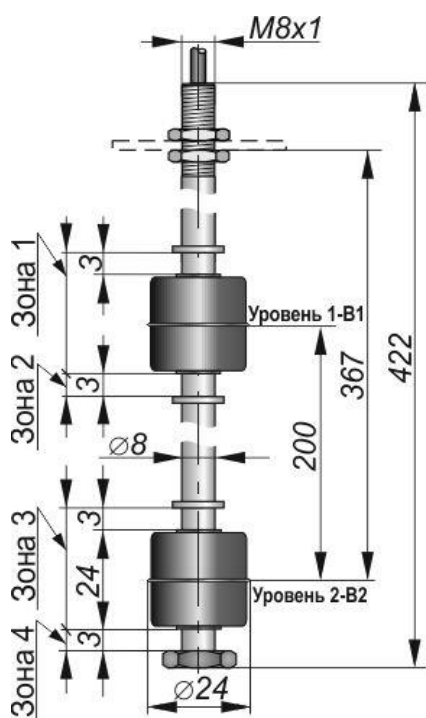
Габаритный чертеж
