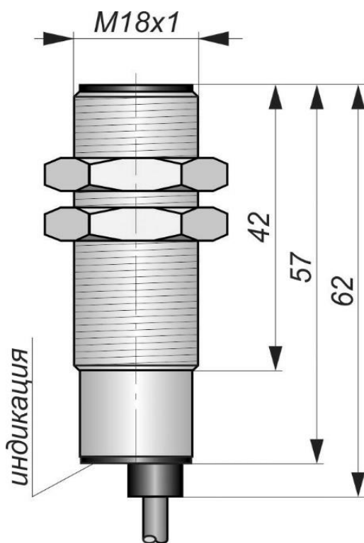
Габаритный чертеж
