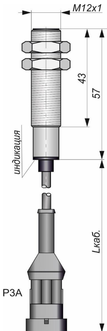
Габаритный чертеж
