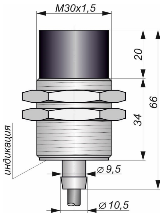
Габаритный чертеж
