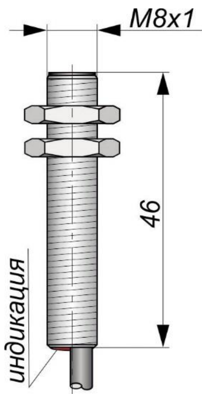
Габаритный чертеж
