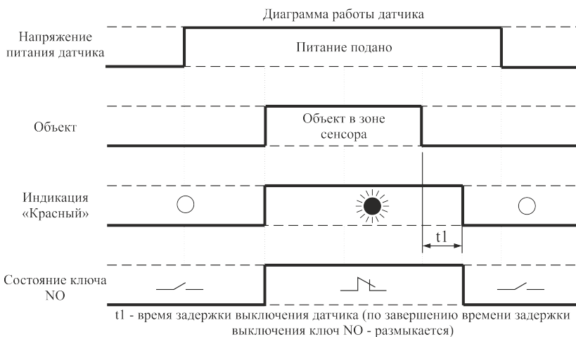
Нормально-разомкнутый контакт
