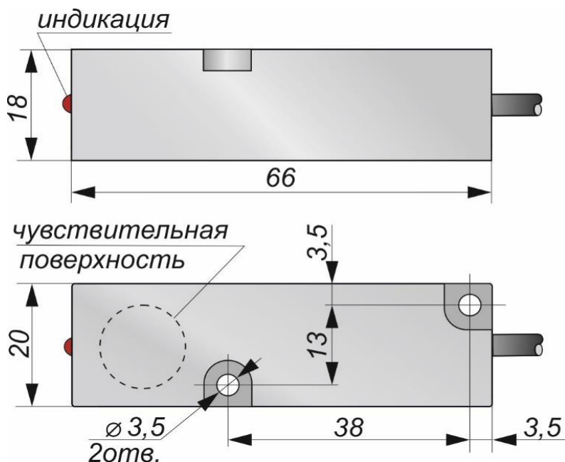
Габаритный чертеж
