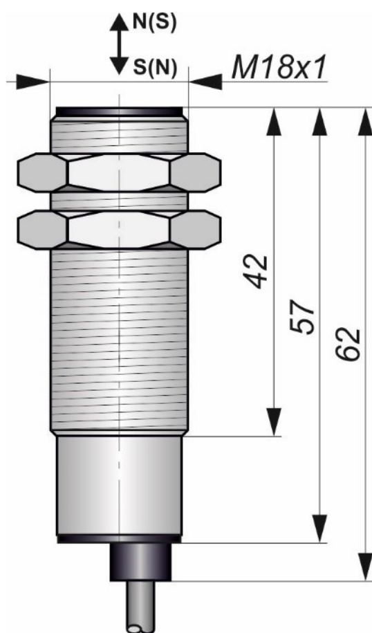
Габаритный чертеж
