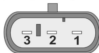
Схема соединения
