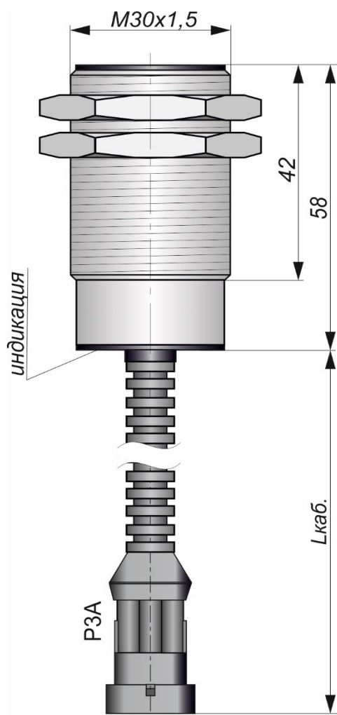
Габаритный чертеж
