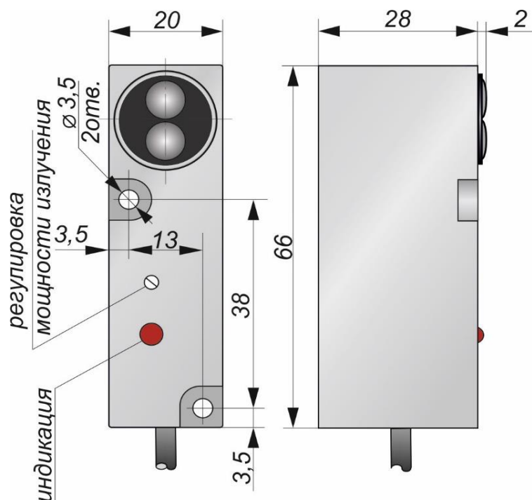
Габаритный чертеж
