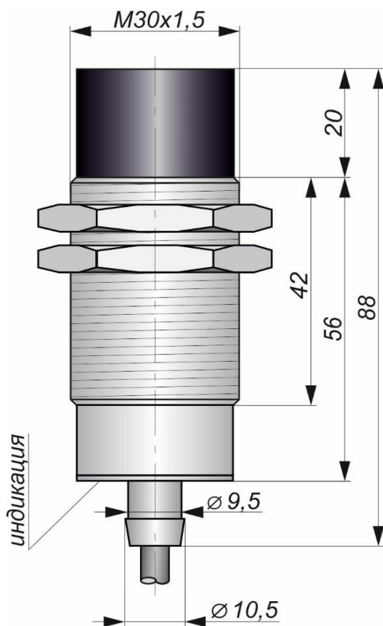
Габаритный чертеж
