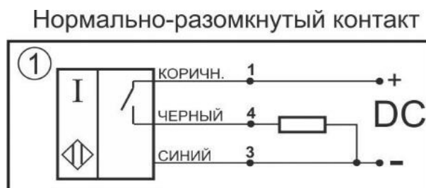
Схема соединения
