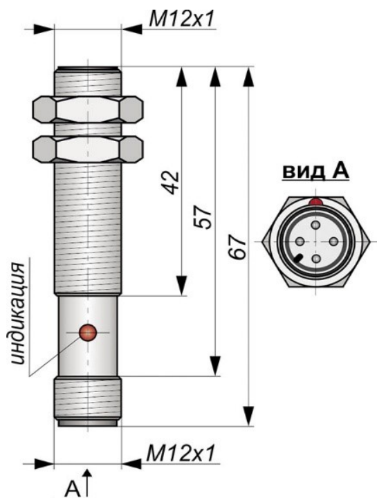
Габаритный чертеж
