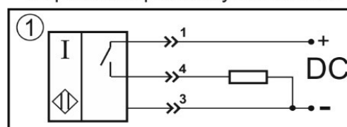
Цоколевка разъема
