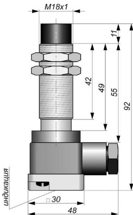
Габаритный чертеж
