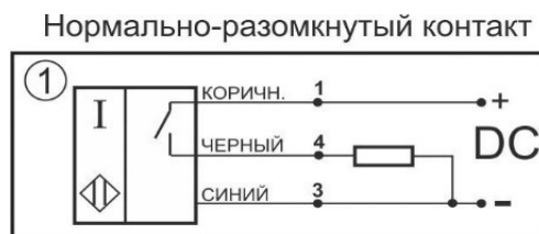
Схема соединения
