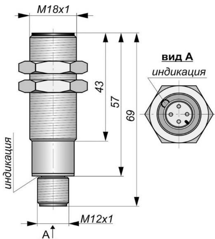
Габаритный чертеж
