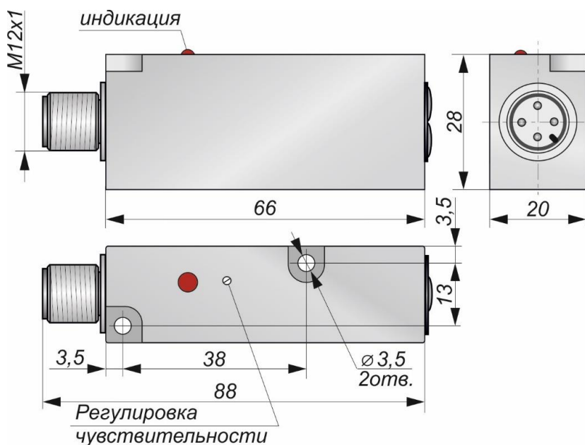
Габаритный чертеж
