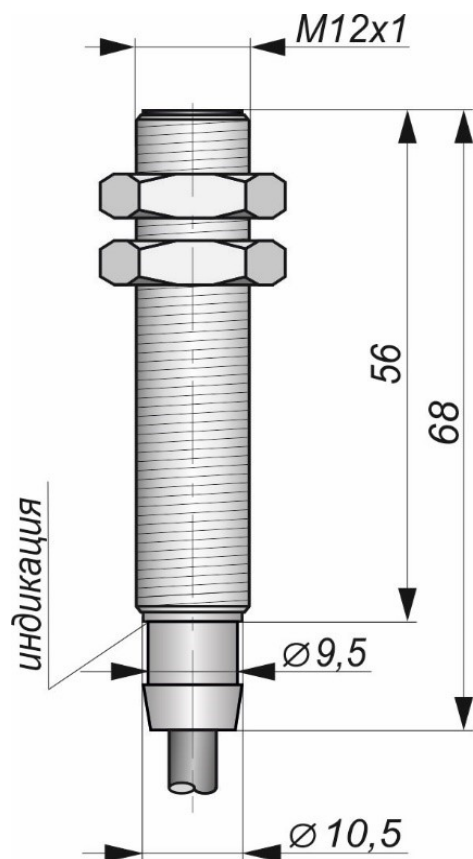
Габаритный чертеж
