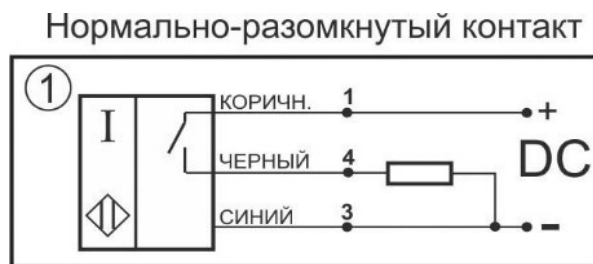
Схема соединения
