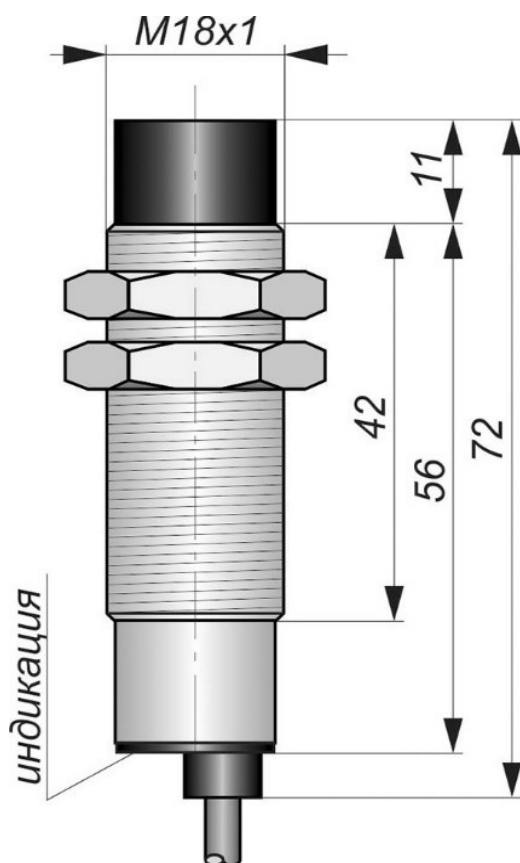
Габаритный чертеж
