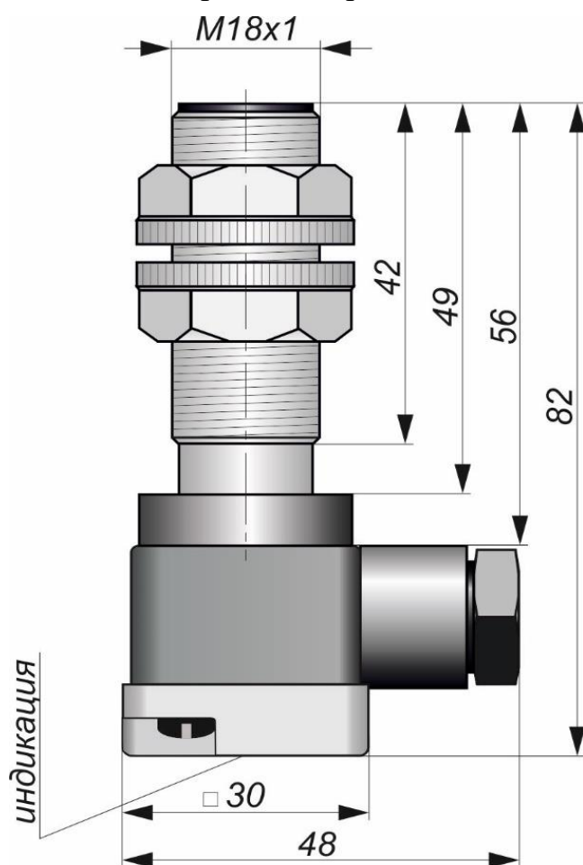
Габаритный чертеж
