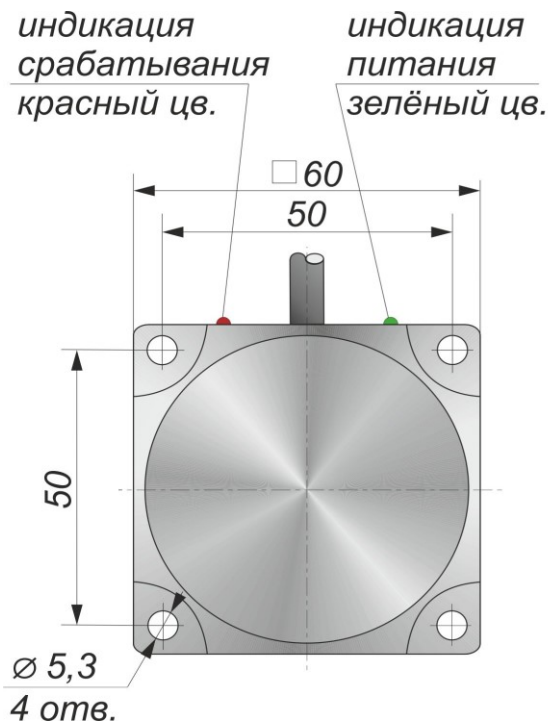
Габаритный чертеж
