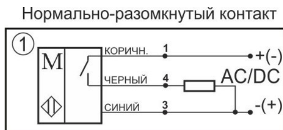
Схема соединения
