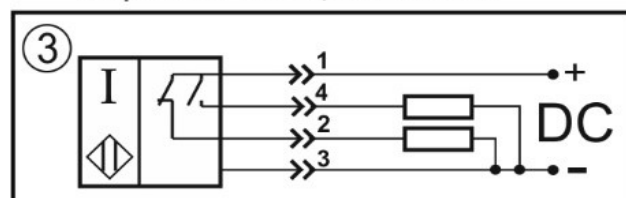
Переключающий контакт
