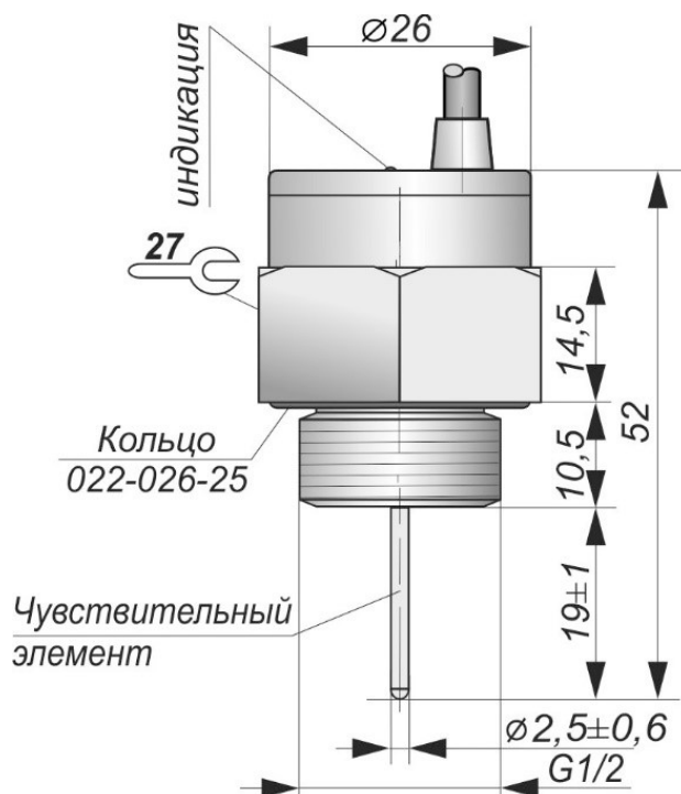
Габаритный чертеж
