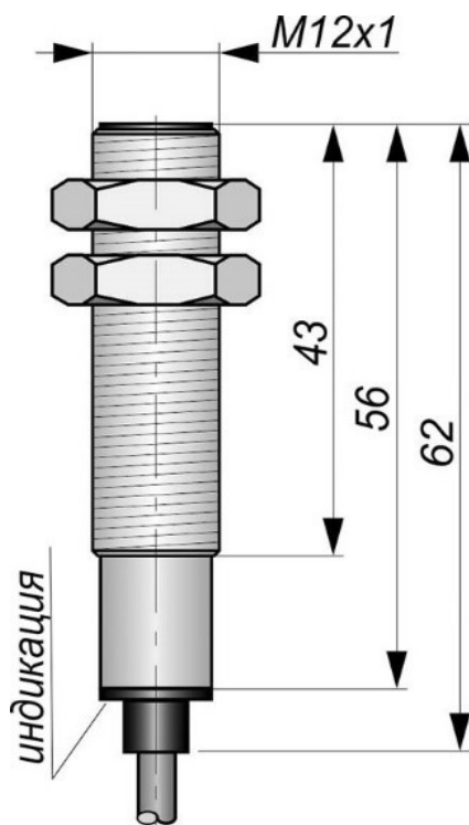
Габаритный чертеж
