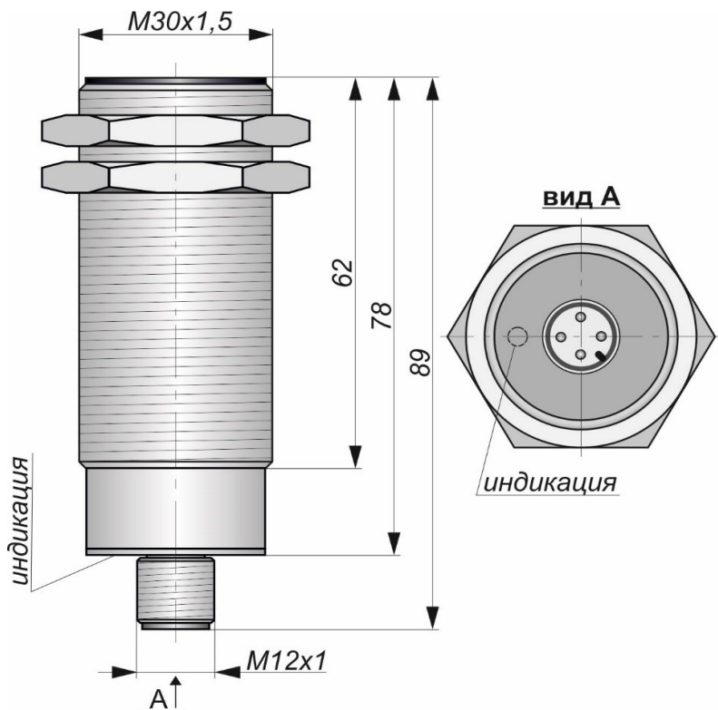
Габаритный чертеж
