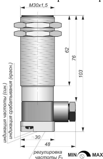
Габаритный чертеж
