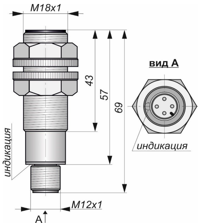
Габаритный чертеж
