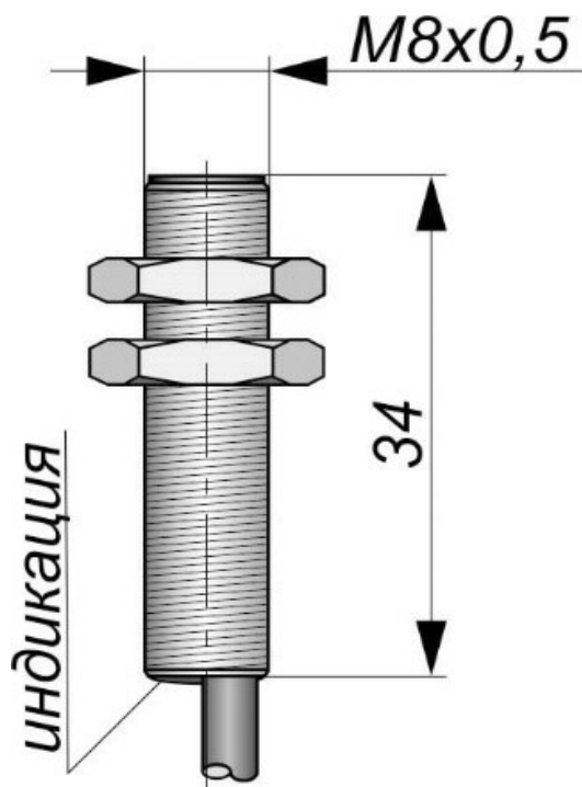
Габаритный чертеж
