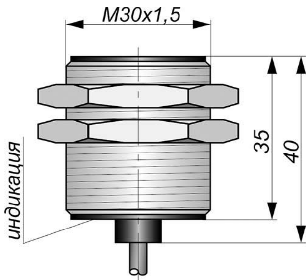
Габаритный чертеж
