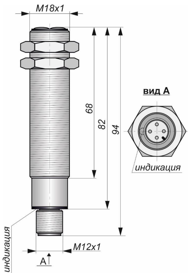
Габаритный чертеж
