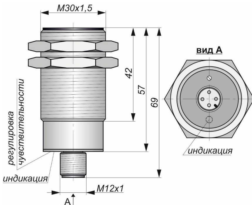
Габаритный чертеж
