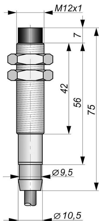
Габаритный чертеж
