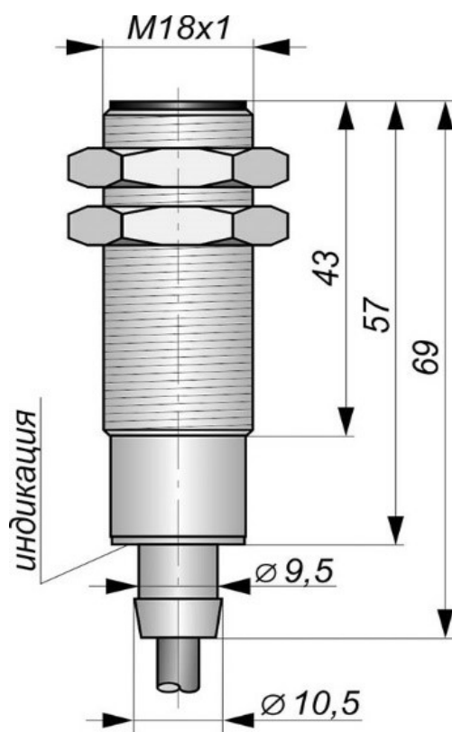
Габаритный чертеж
