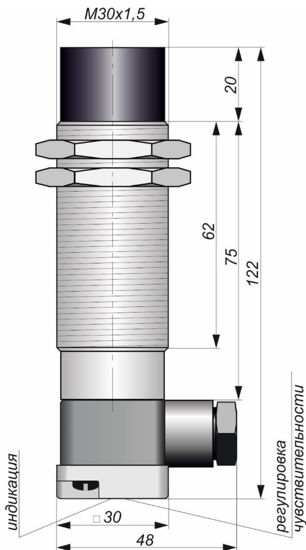
Габаритный чертеж
