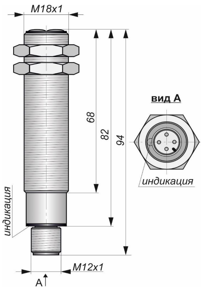
Габаритный чертеж
